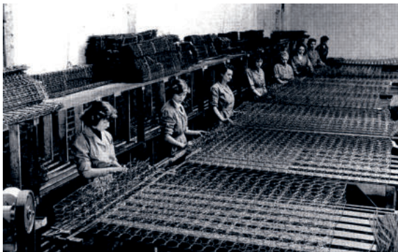
Manuelle Montage von Pullman-Federung
